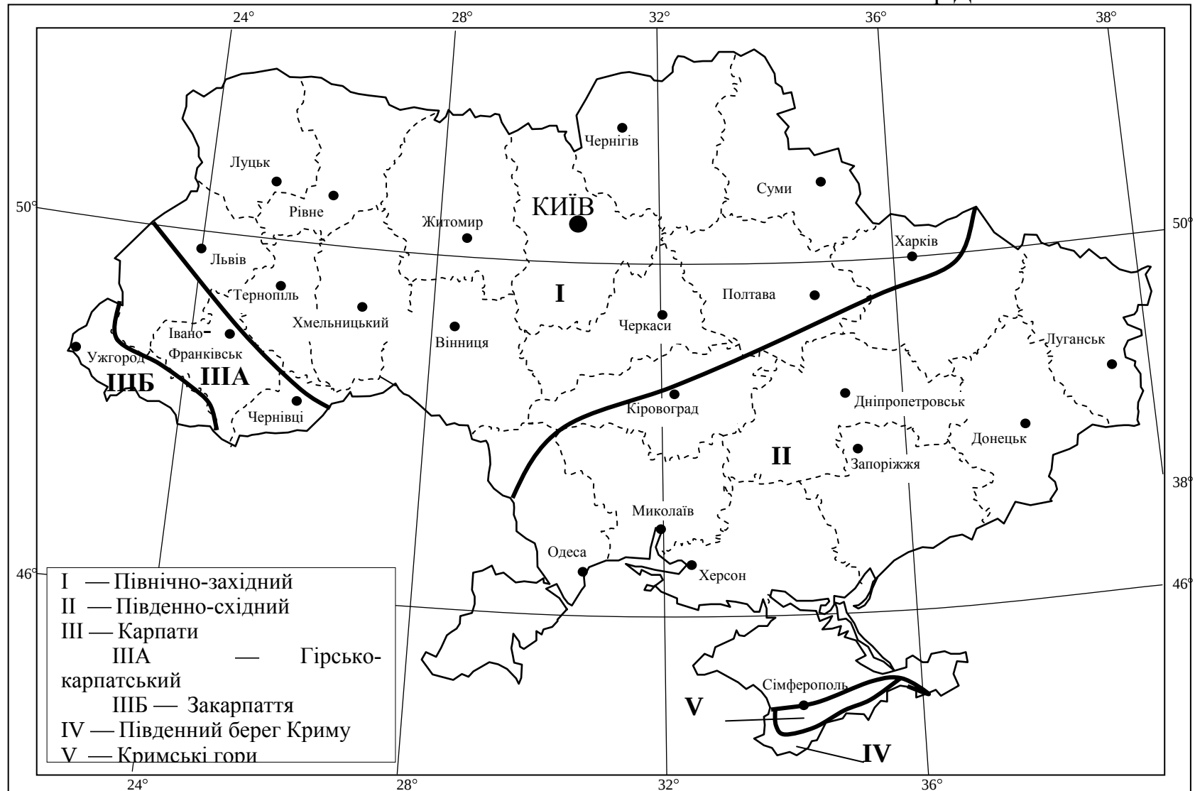
Рисунок 1 – Архітектурно-будівельне кліматичне районування території України
