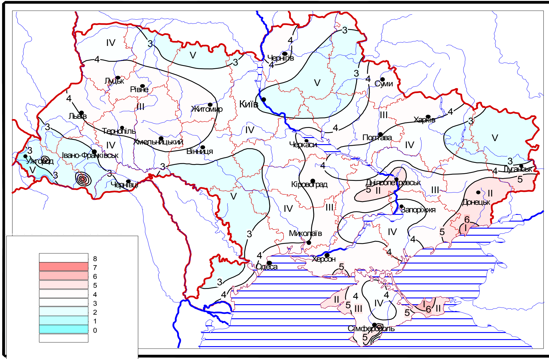
Рисунок 3 – Районування України за середньою швидкістю вітру, м/с, в січні:
